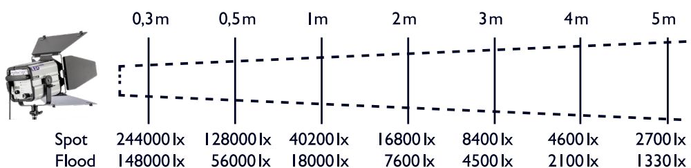
Leistungsdiagramm / performance chart
